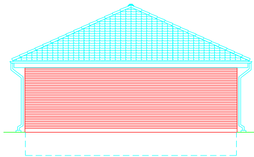
Vestfacade 1:100
