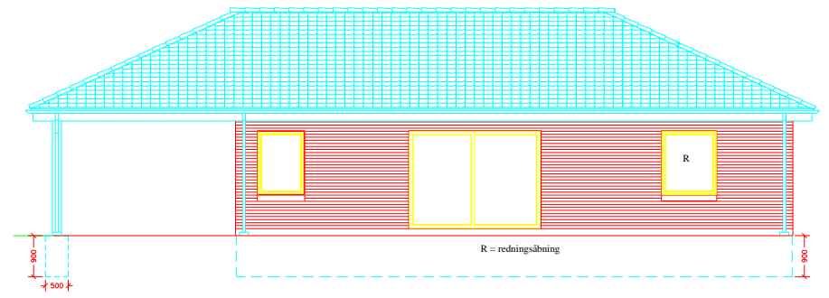
Nordfacade 1:100
