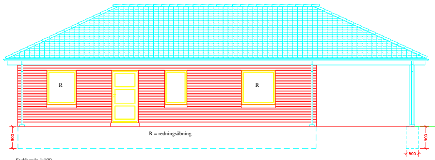
Sydfacade 1:100
